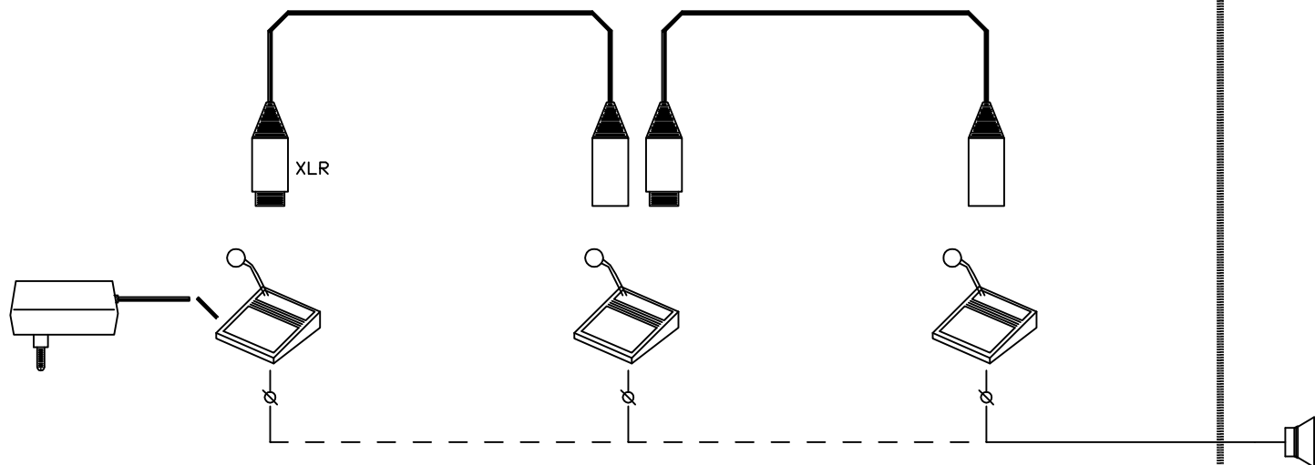
3 MIKROFONOVE TERMINALY SPOJENE PARTY-LINE ZBERNICOU
